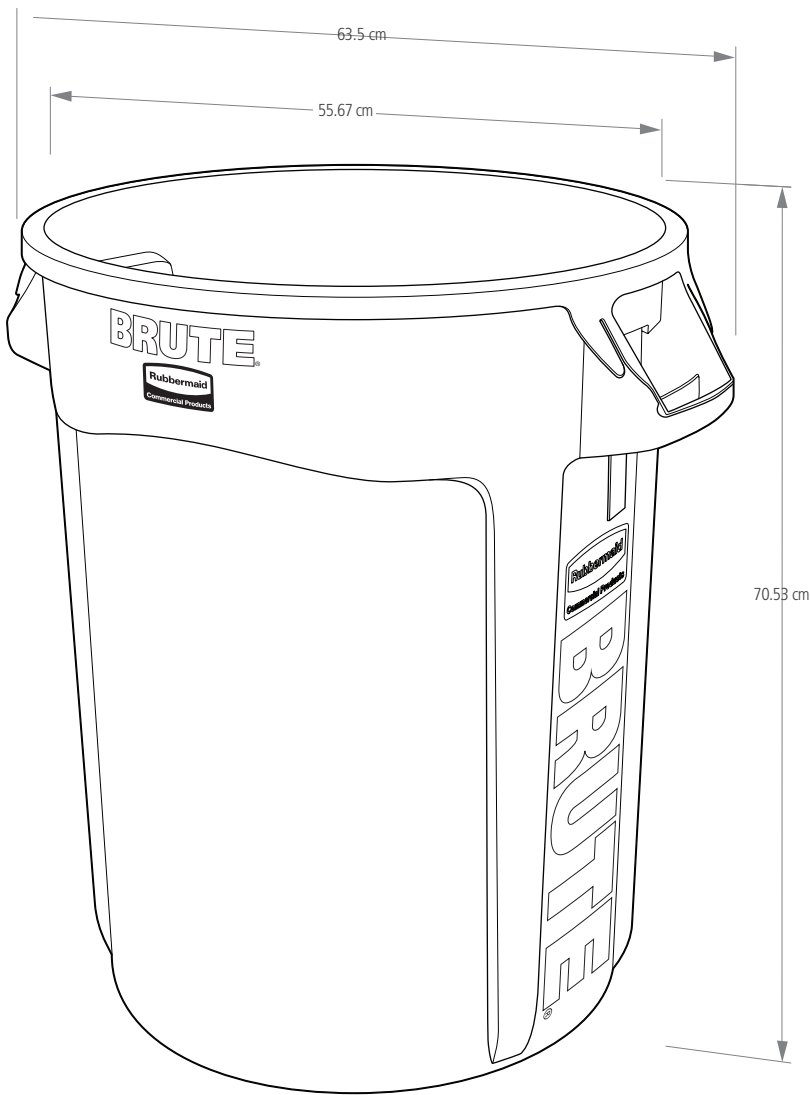
Contenedor 121 L
